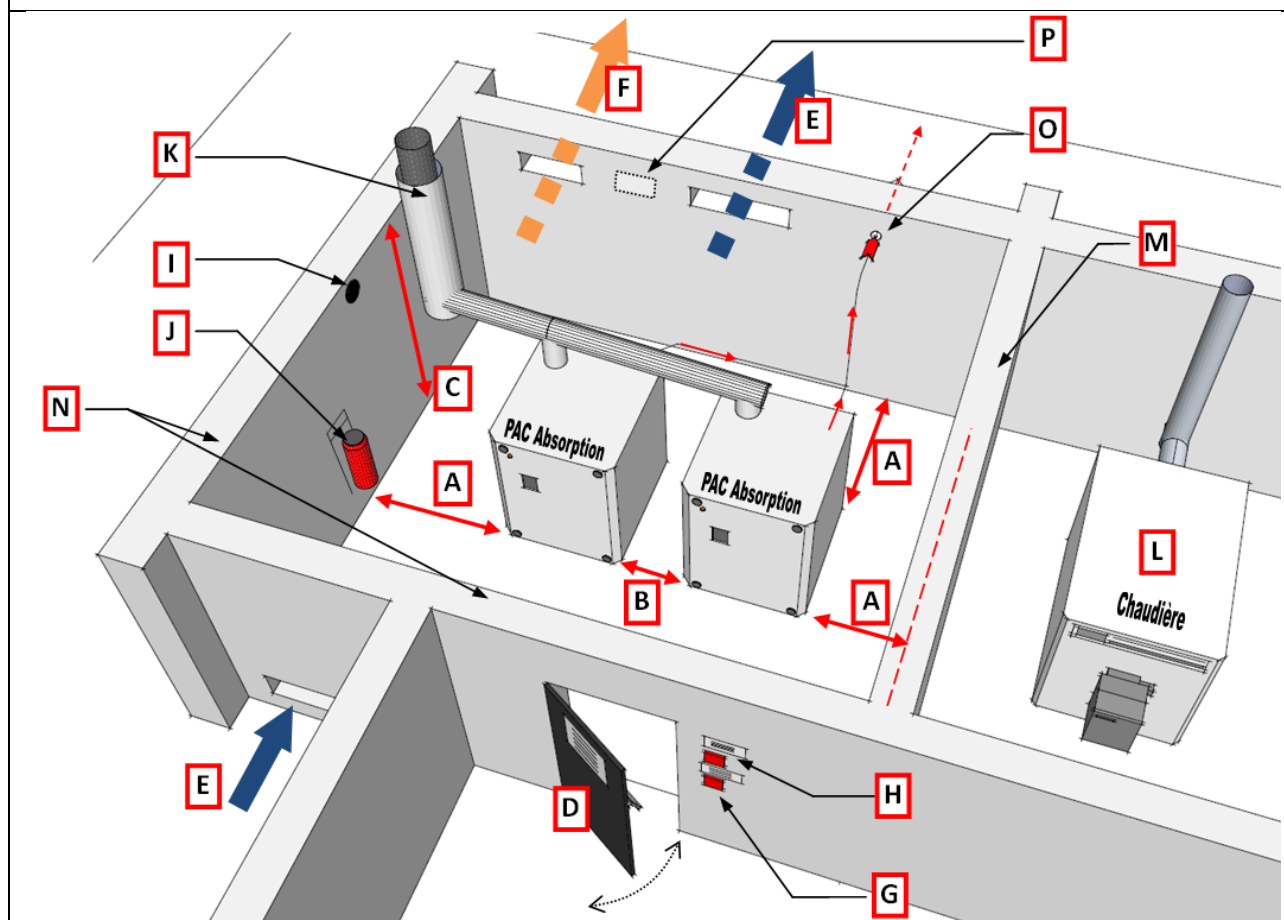
Figure 2.1 : Exemple d'implantation d'une salle des machines
